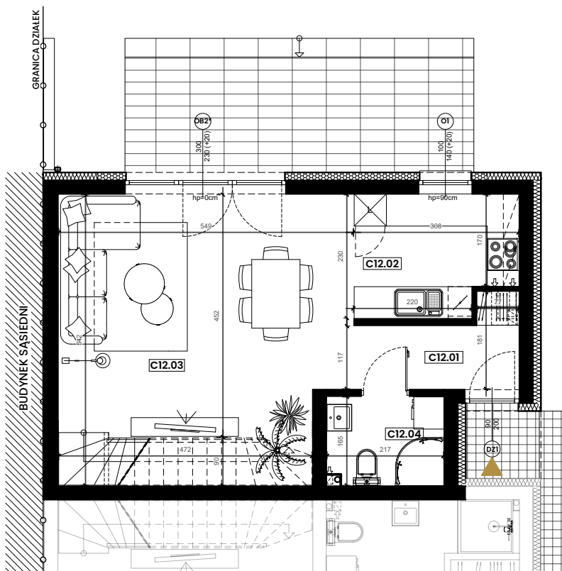
RZUT PARTERU
