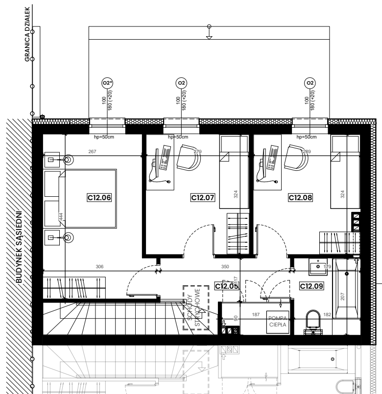
RZUT PIĘTRA
