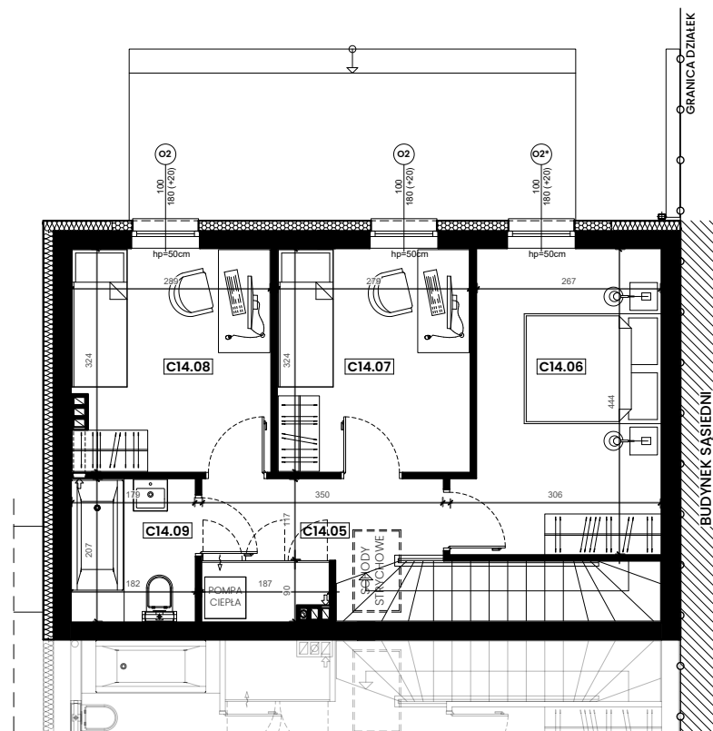
RZUT PIĘTRA
