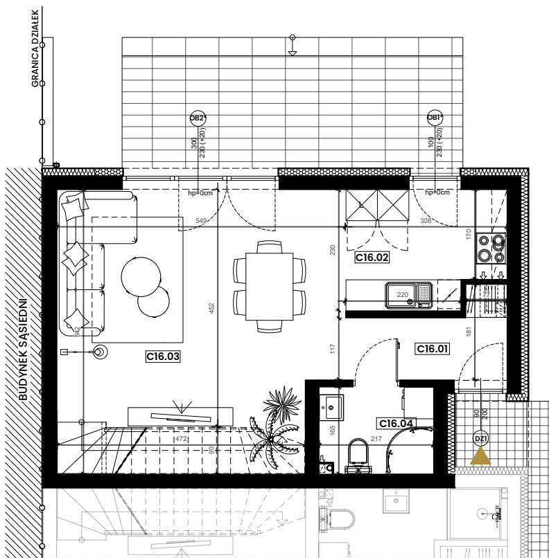
RZUT PARTERU
