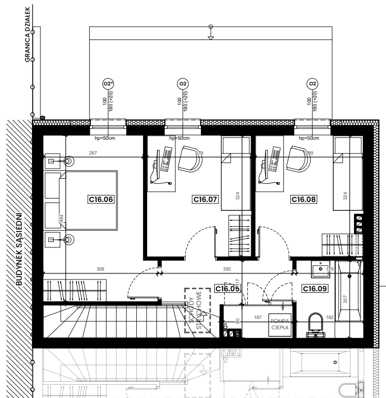
RZUT PIĘTRA
