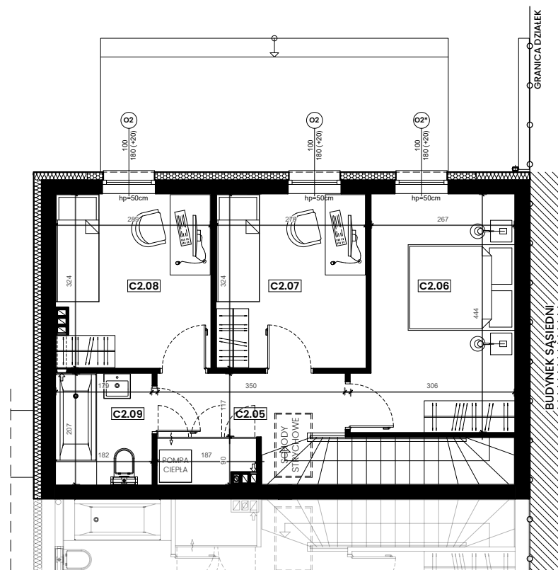
RZUT PIĘTRA
