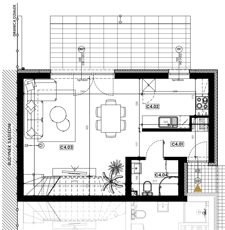
RZUT PARTERU
