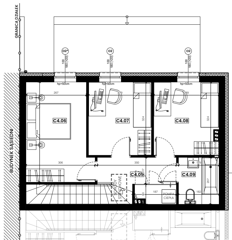
RZUT PIĘTRA
