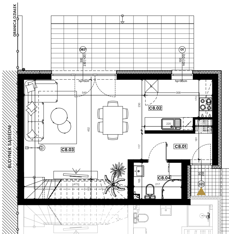
RZUT PARTERU
